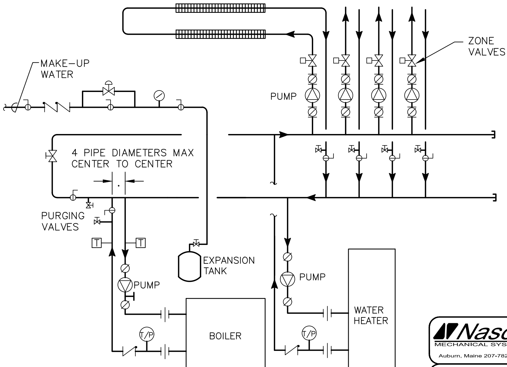
BOILER PRIMARY DETAIL N.T.S.
